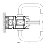
Door lock
